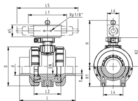
DN65-100
