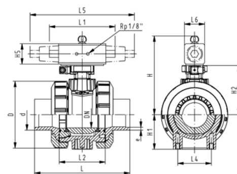
DN65-100
